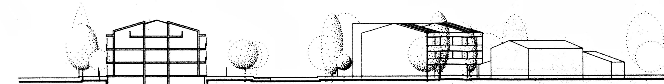
SEZIONE B-B scala 1:500
