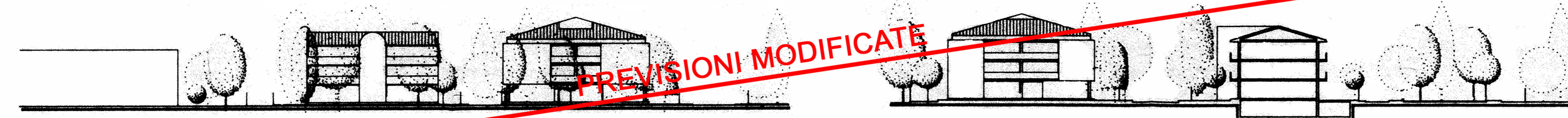
PROSPETTO LATO SUD EST VIA DEGLI STAGNACCI LOTTO 12 scala 1:500 SEZIONE C-C SCALA 1:500
